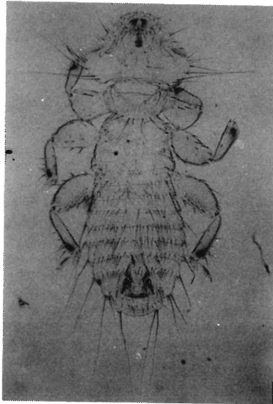
Abb. 2: Myrsidea pilosa ♂
