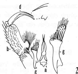
Orimarga ( Orimarga ) frommeri sp. n. Fig. 1. Venation
